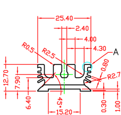
SCALE 5:1
